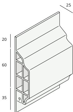
Dakrandsierprofiel nr. 2110
