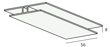
Verbindingprofiel nr. 2284
