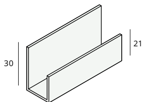
Omrandingprofiel nr. 2120
