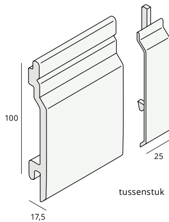
Sponningdeel nr. 2117
