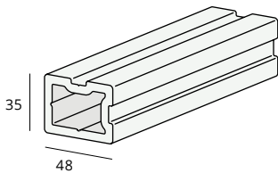
Montageprofiel nr. 2957
