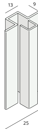
Omegaprofiel nr. 1830
