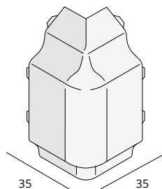
Hoekstuk nr. 2111
