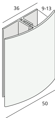
Verbindingsprofiel nr. 0409
