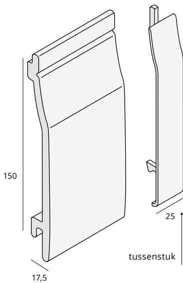
Rabatdeel nr. 2115
